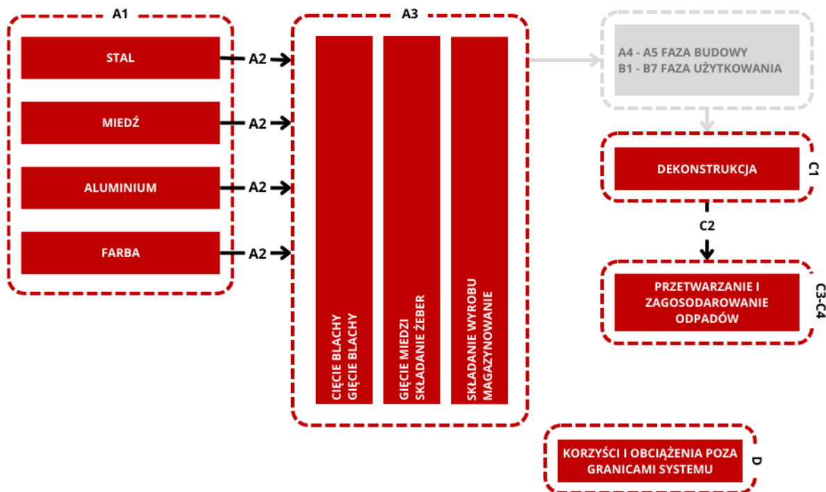
Rysunek 5.1: Granice systemu wykorzystane do charakterystyki środowiskowej grzejników kanałowych
